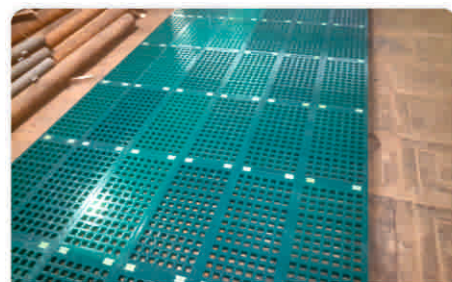
Сита полиуретановые на подситнике
