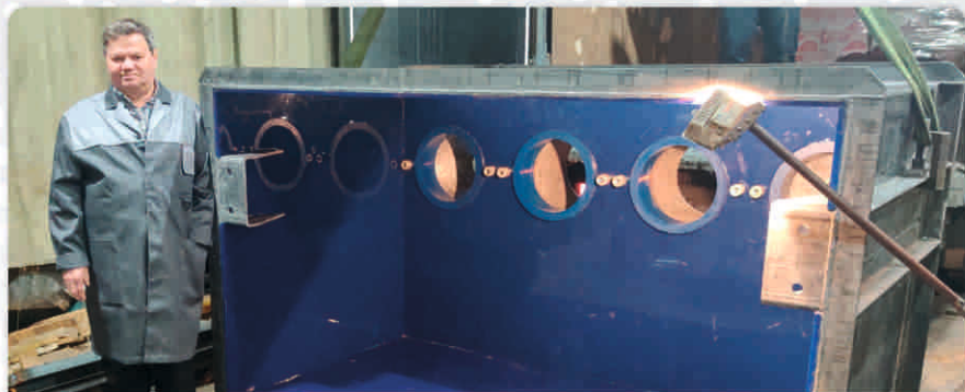
Короб пульподелителя футерованный полиуретаном
